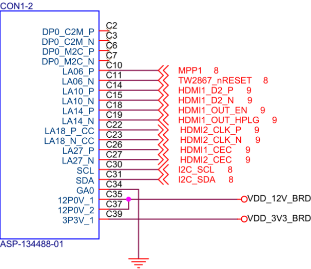
图 7 FMC 连接器引脚定义 1
