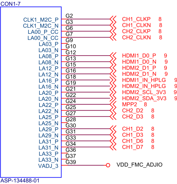
图 9 FMC 连接器引脚定义 3
