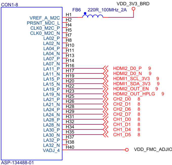
图 10 FMC 连接器引脚定义 4
