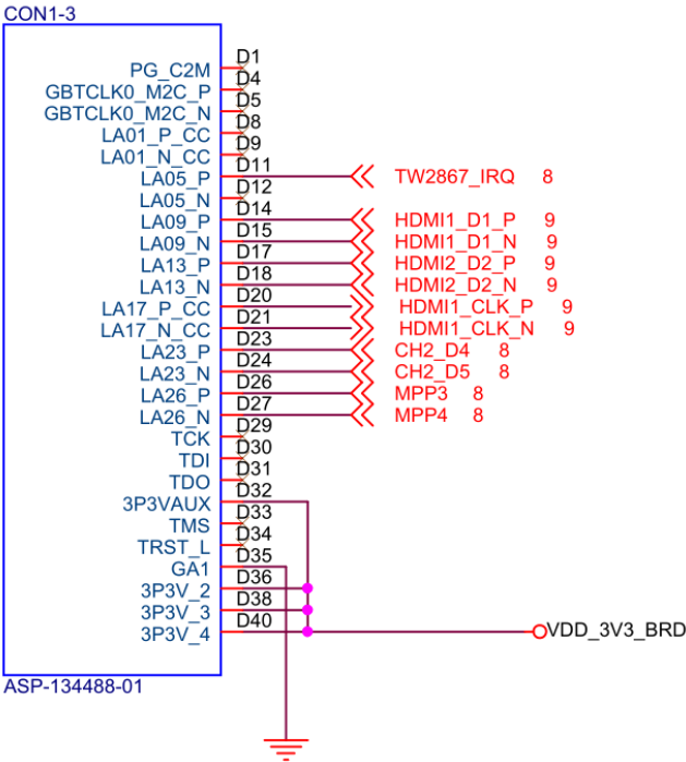
图 8 FMC 连接器引脚定义 2
