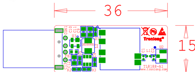
图 3 模块机械尺寸图
