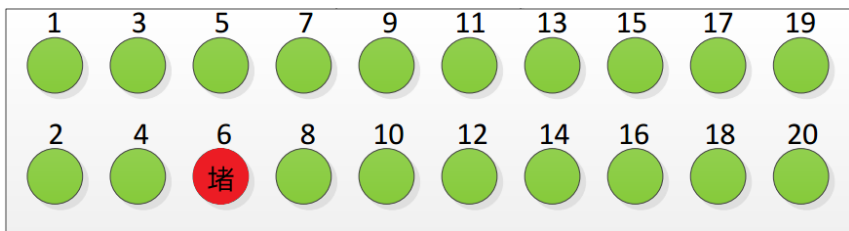
图 5 20pin JTAG 转接头引脚位置示意图
