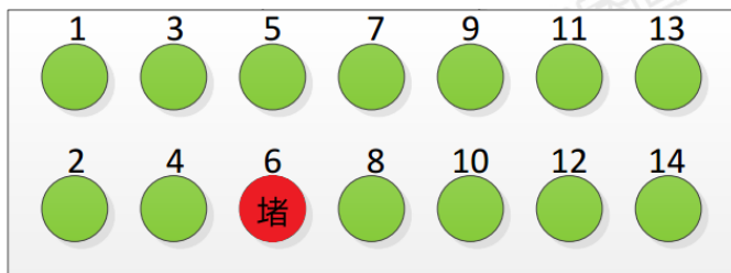
图 6 14pin JTAG 转接头引脚位置示意图
