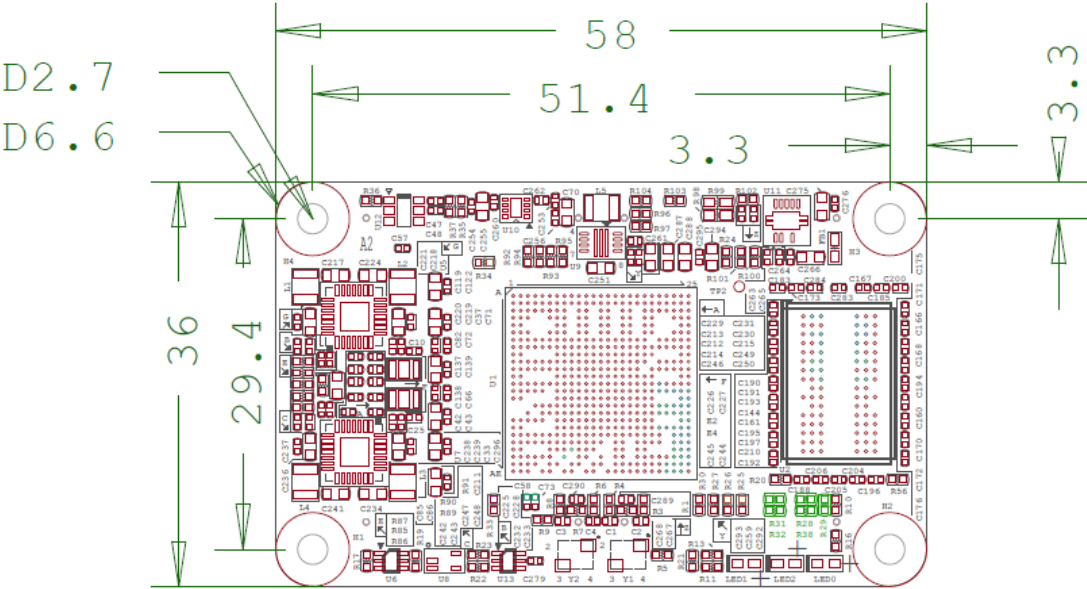
图 11 核心板机械尺寸图
