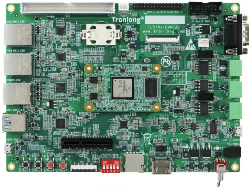
图 1 评估板正面图 1
