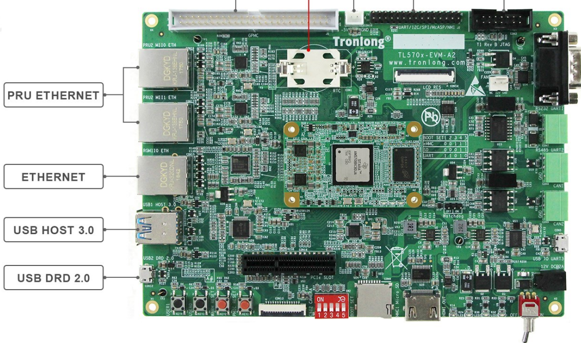
图 9 评估板硬件资源图解 1
