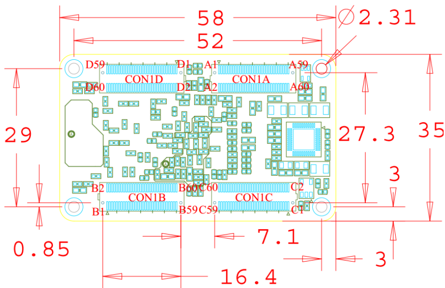
图 10 核心板机械尺寸图
