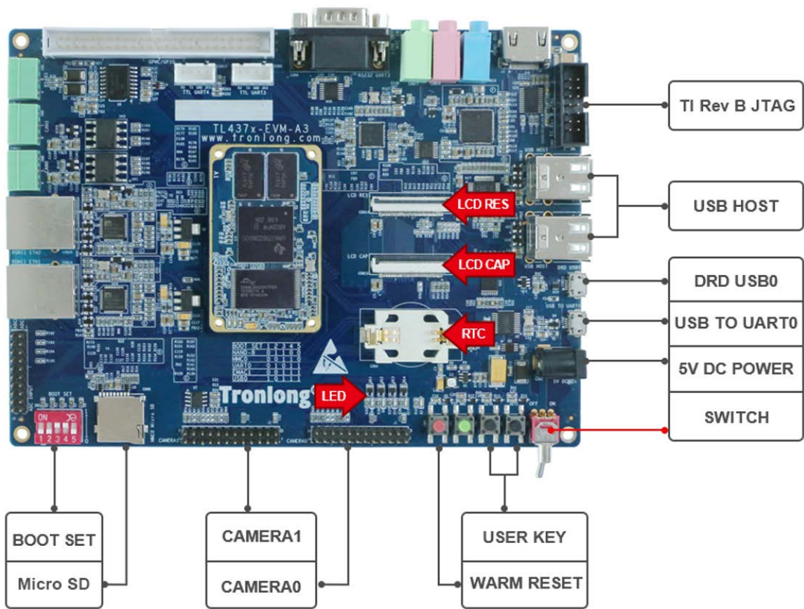
图 9 评估板硬件资源图解 2
