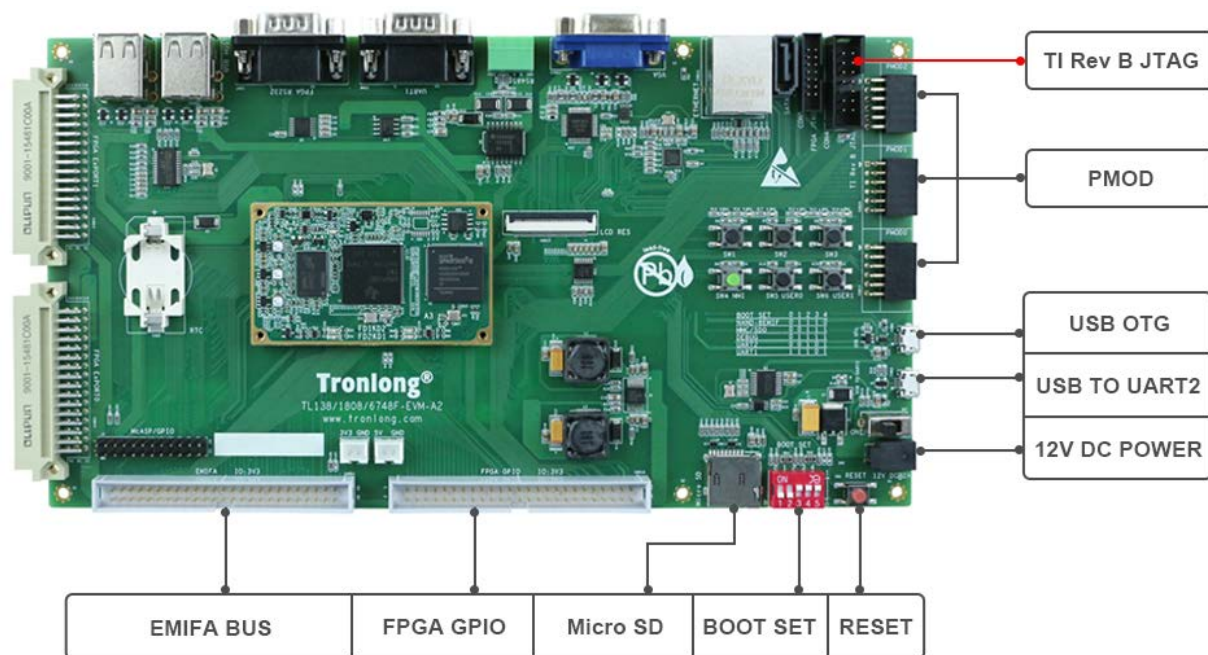
图 10 开发板硬件资源图解 2
