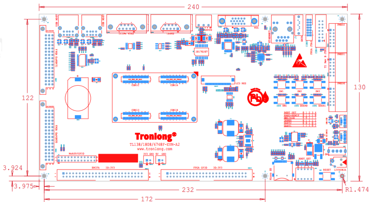
图 13 开发板底板机械尺寸图
