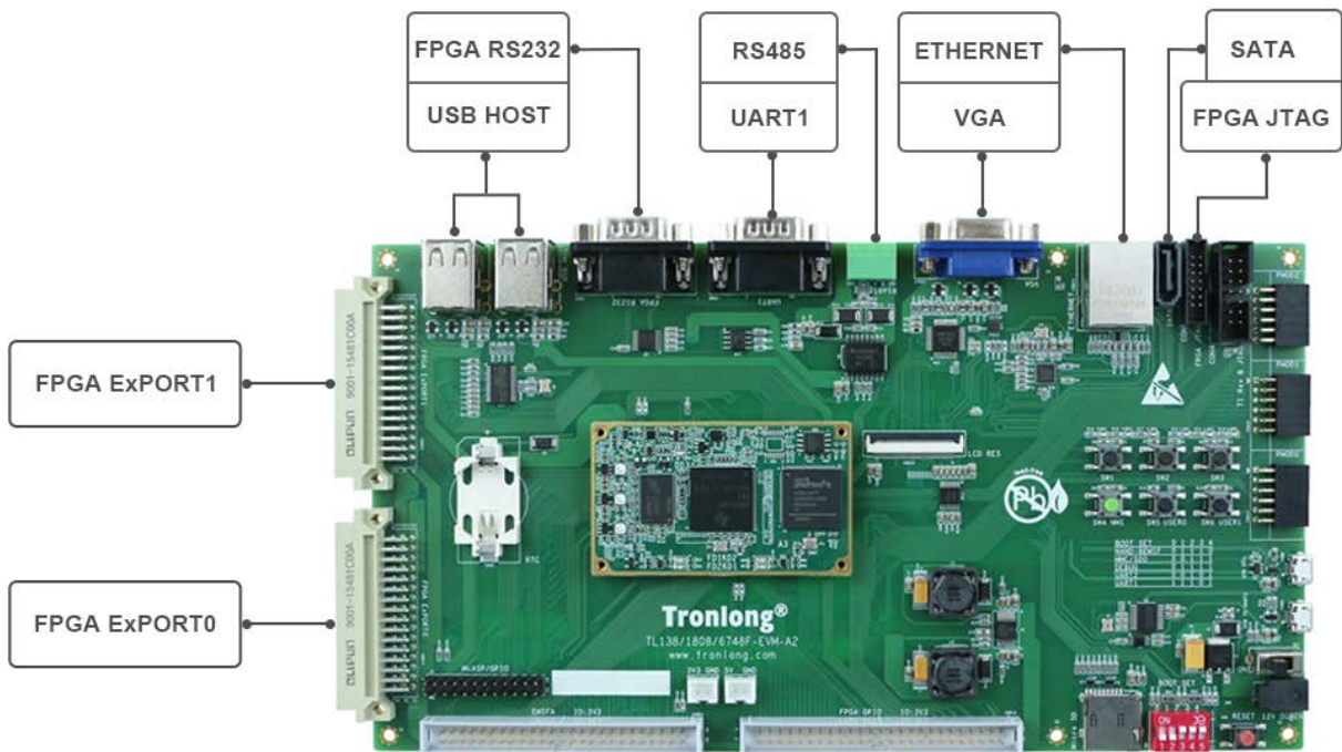
图 9 开发板硬件资源图解 1
