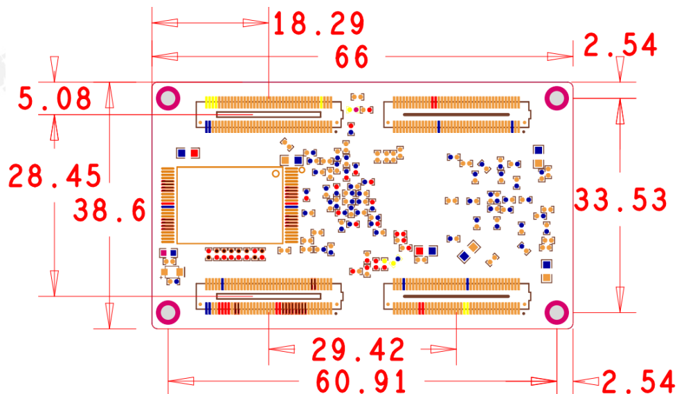
图 12 核心板机械尺寸图
