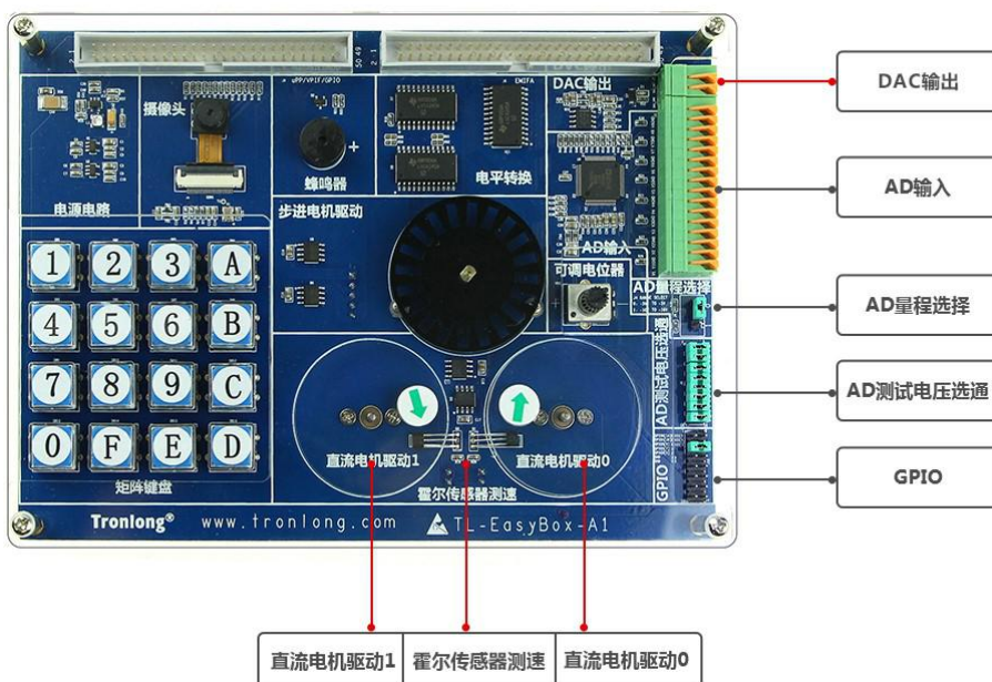
图 11 实验拓展板硬件资源图解 2
