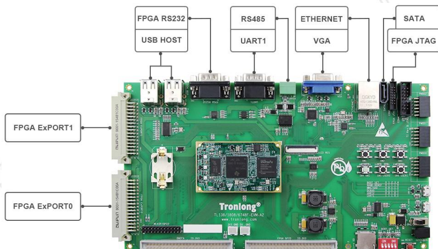
图 8 实验主板硬件资源图解 1
