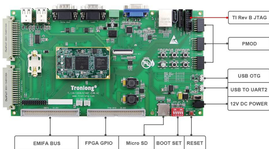
图 9 实验主板硬件资源图解 2
